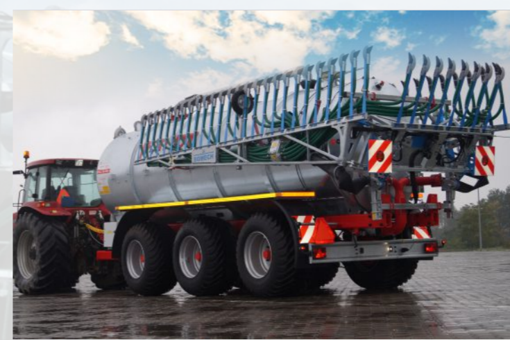
APLIKATORY typ łyżwy wleczone
